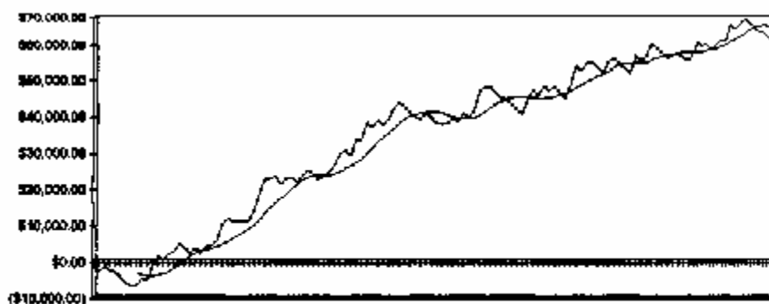
Рис. 11.1 Кривая, которая получается, если заключать сделки сразу после падения цены ниже средней капитала.
